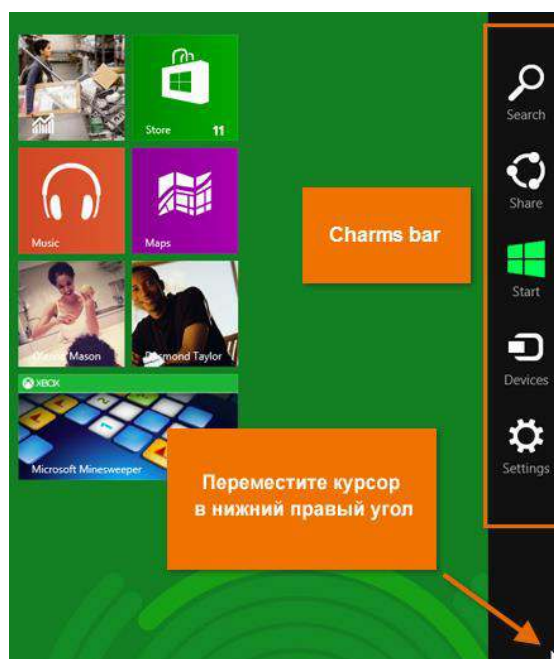
Рис. 4 – Всплывающая панель.
